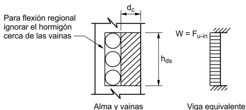
Figura C 5.10.4.3.1c-1. Recubrimiento de hormigón de una viga hipotética sin armar
