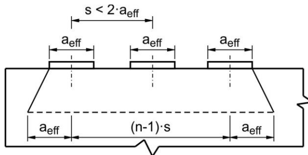
Figura C 5.10.9.6.2-2. Múltiples anclajes poco separados
