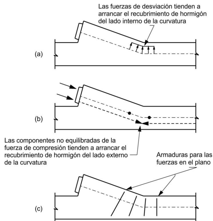
Figura C 5.10.4.3.1a-1. Fuerzas en el plano en un taco para anclaje
