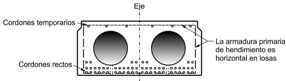
Figura C 5.10.10.1-2. Losa hueca prefabricada
