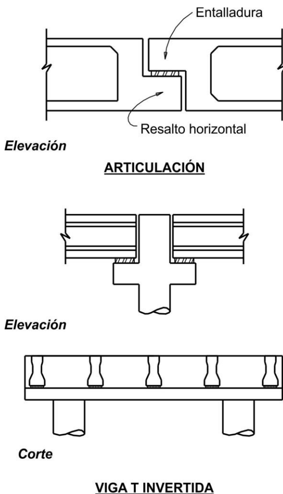
Figura C 5.13.2.5.1-1. Ejemplos de vigas con resaltos horizontales
