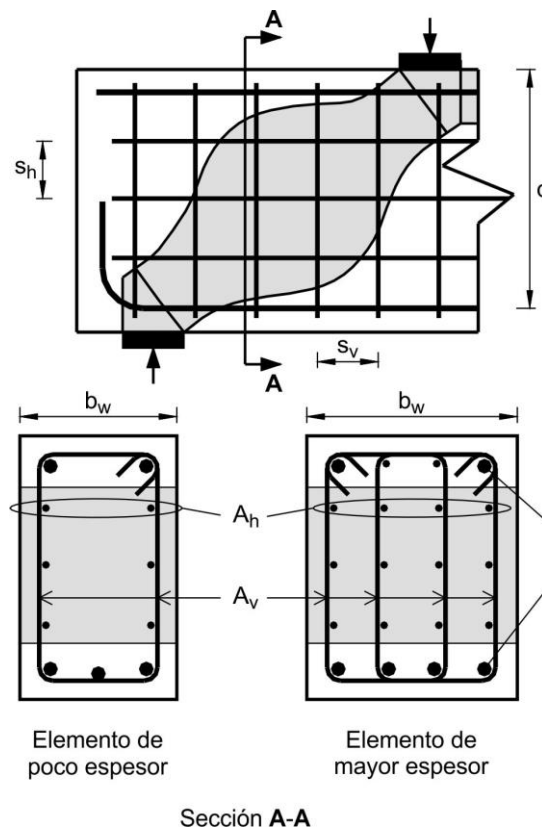
Figura C 5.6.3.6-1. Distribución de la armadura para limitar la fisuración en una biela comprimida
