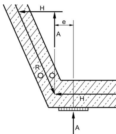
Figura C 5.14.2.4.6c-2. Reacción excéntrica en las placas de lanzamiento
