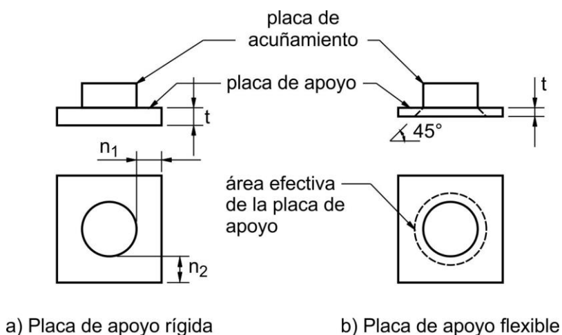
Figura C 5.10.9.7.2-2. Área efectiva de la placa de apoyo para dispositivos de anclaje con placa de acuñaamiento separada
