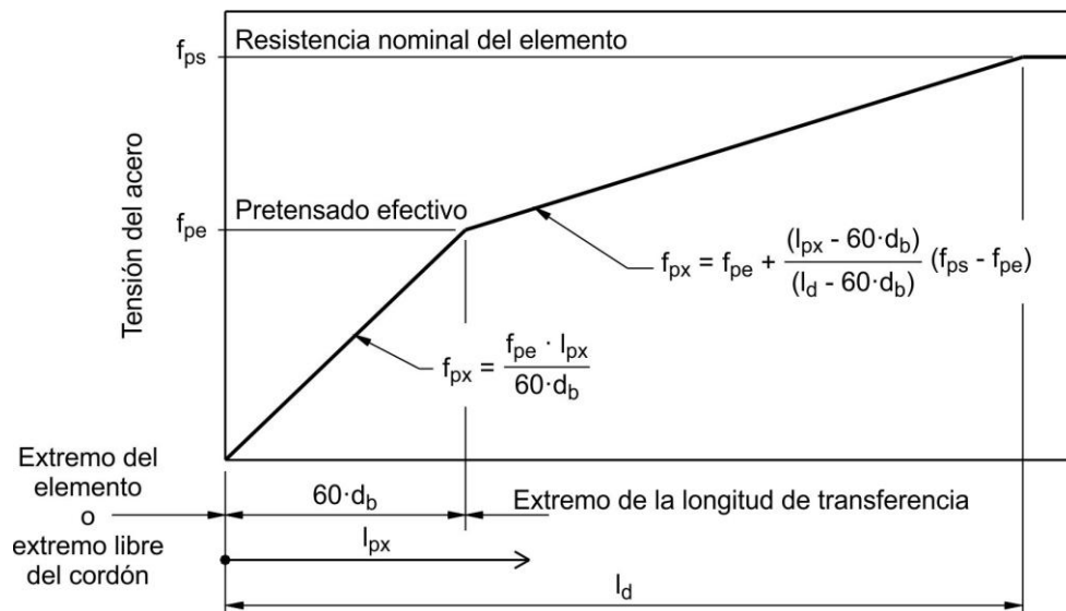
Figura C 5.11.4.2-1. Relación teórica entre la tensión del acero y la distancia desde el extremo libre del cordón.
