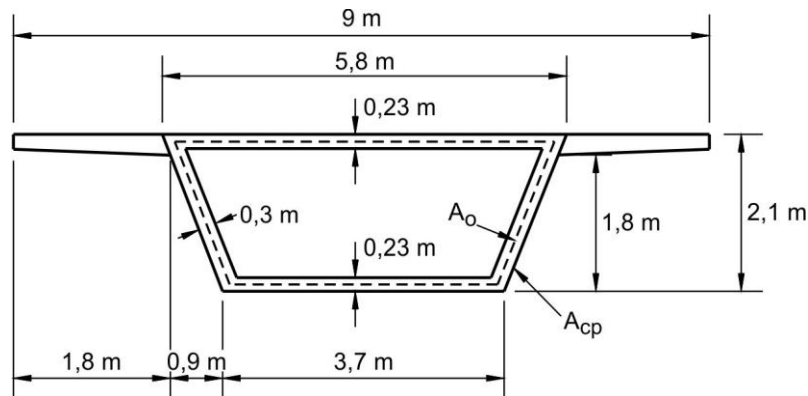
Figura C 5.8.2.1-1. Esquema que muestra los datos usados en el ejemplo de cálculo de A_o incluido a continuación
