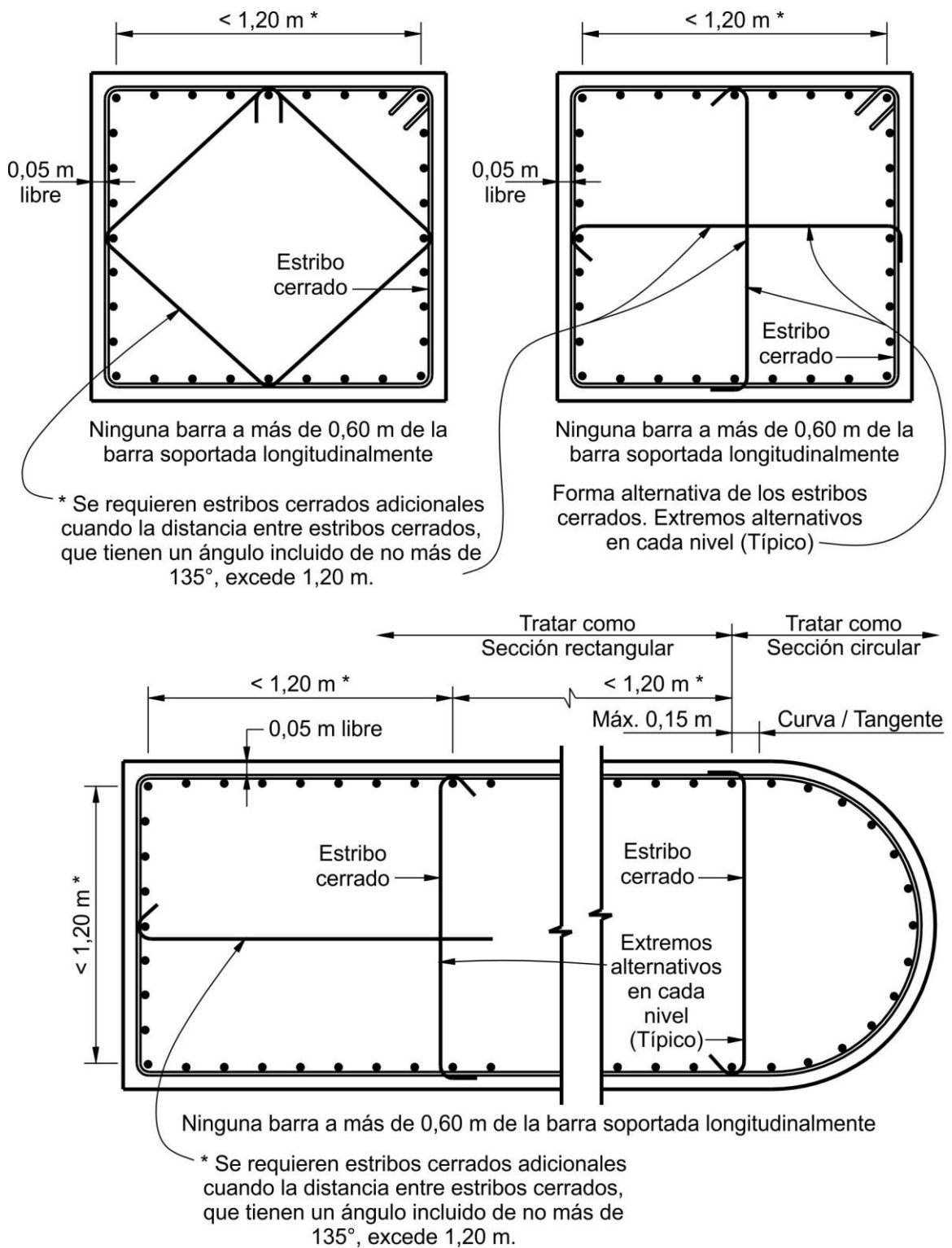
Figura C 5.10.6.3-1. Armado aceptable de los estribos cerrados
