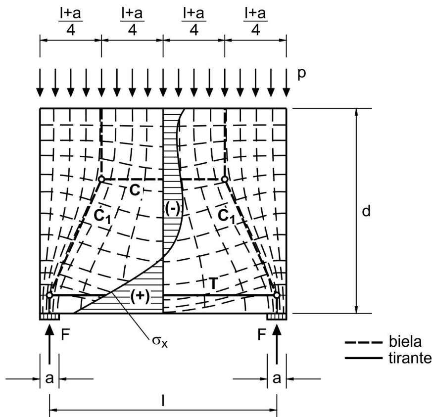
Figura C 5.10.9.4.1-1. Campo de tensiones principales, y superpuesto con el modelo de bielas y tirantes
