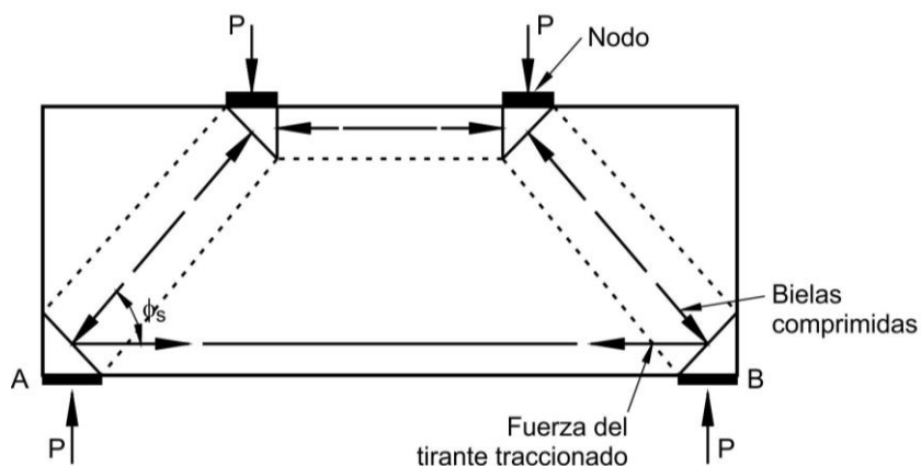
(C) Modelo reticulado
