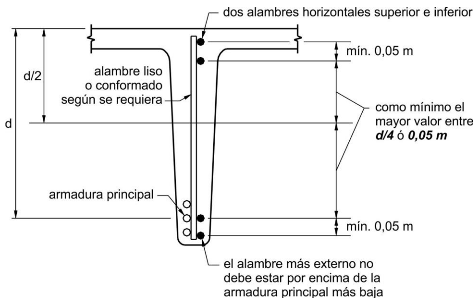
Figura C 5.11.2.6.3-1. Anclaje de la armadura de corte compuesta por un estribo de una rama realizado con malla de acero soldada.
