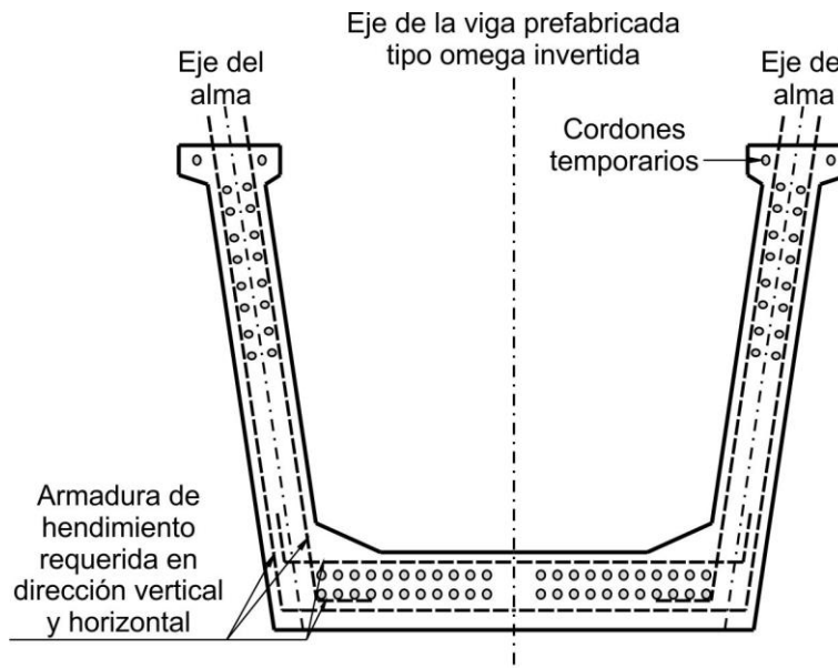
Figura C 5.10.10.1-1. Viga tipo omega invertida prefabricada
