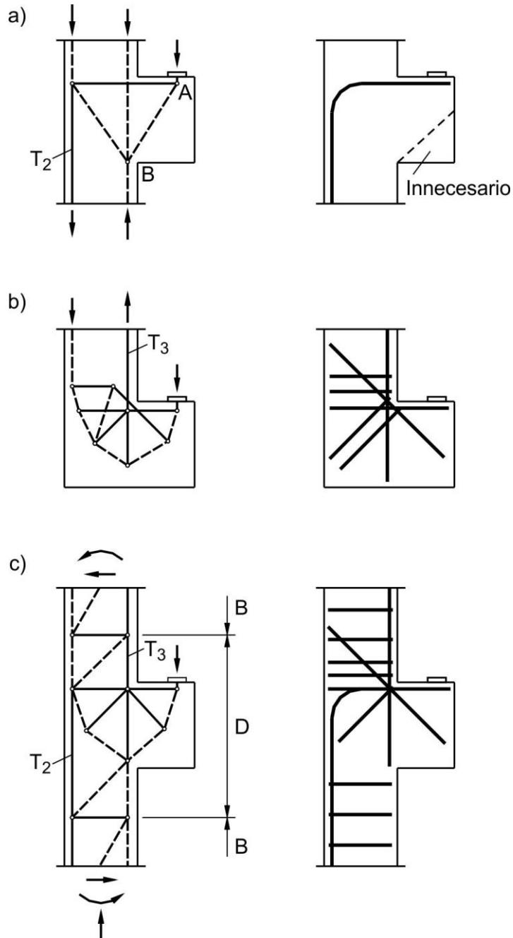
Figura C 5.13.2.4.1-1. Diferentes condiciones de apoyo que conducen a diferentes modelos de bielas y tirantes y diferentes disposiciones de armadura en ménsulas cortas y vigas con resaltes horizontales (Schlaich et al., 1987)
