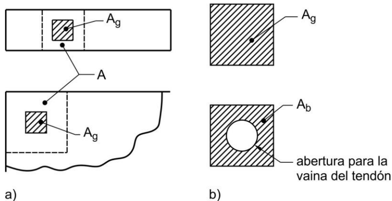
Figura C 5.10.9.7.2-1. Área de la superficie de apoyo de hormigón para la expresión 5.10.9.7.2-2
