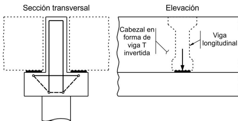
Figura C 5.8.3.2-3. Cabezal consistente en una viga T invertida
