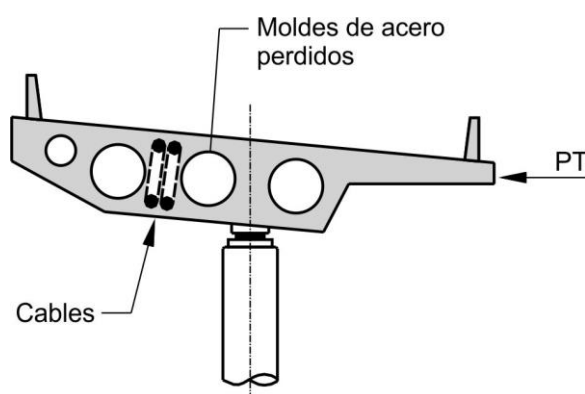
Figura C 5.14.4.2.1-1. Sección transversal de un típico sistema de tablero aligerado
