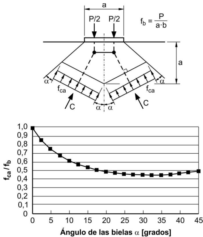
Figura C 5.10.9.6.2-1. Zona local e interfase de las bielas
