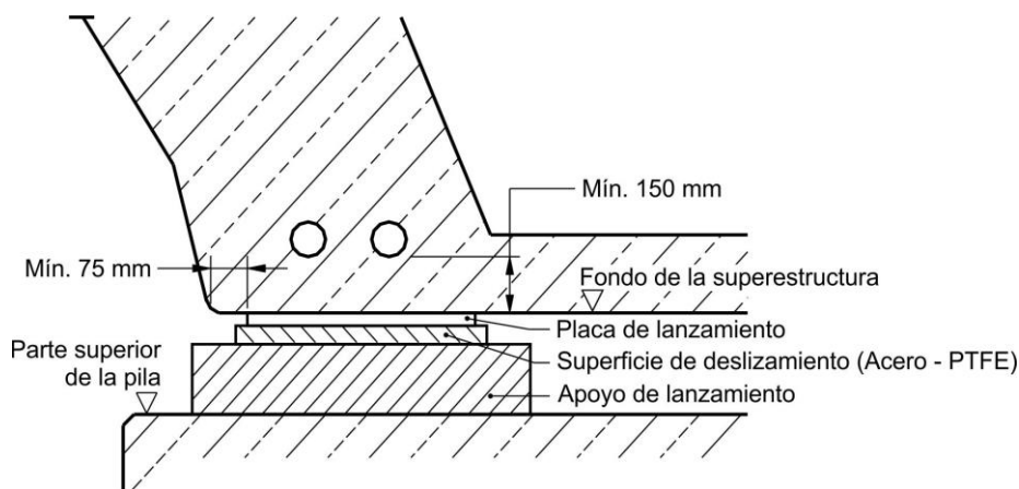
Figura C 5.14.2.4.6c-1. Ubicación de las placas de lanzamiento
