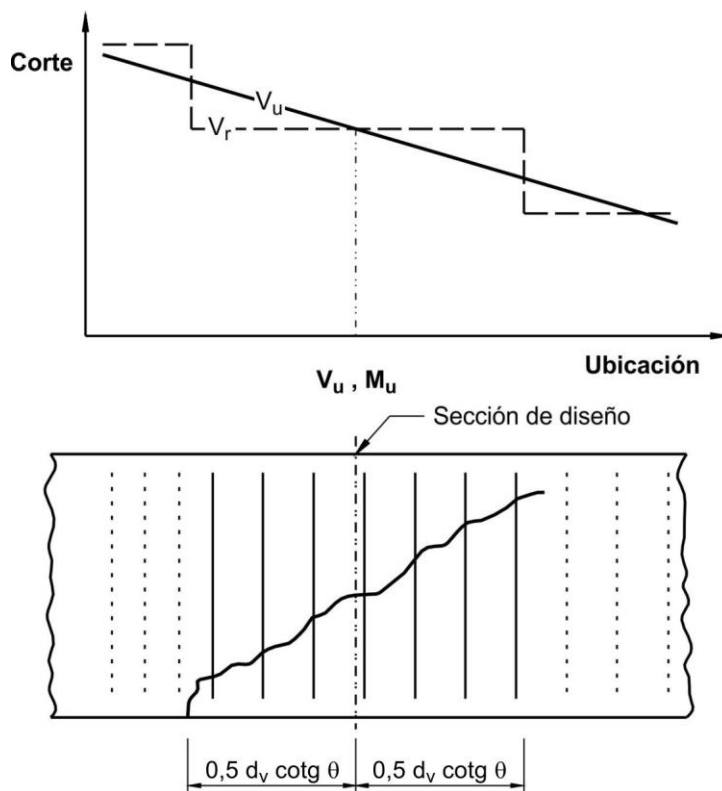
Figura C 5.8.3.2-2. Sección para el diseño simplificado en el caso de cargas aplicadas a la mitad de la profundidad del elemento o por encima de la misma
