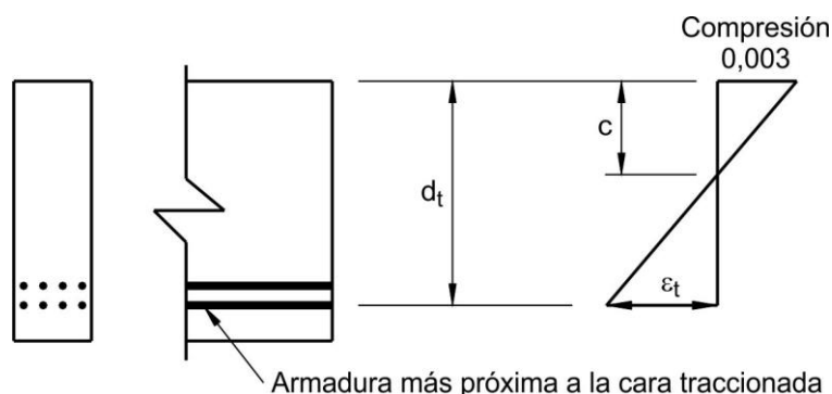
Figura C 5.7.2.1-1. Distribución de las deformaciones y deformación neta por tracción
