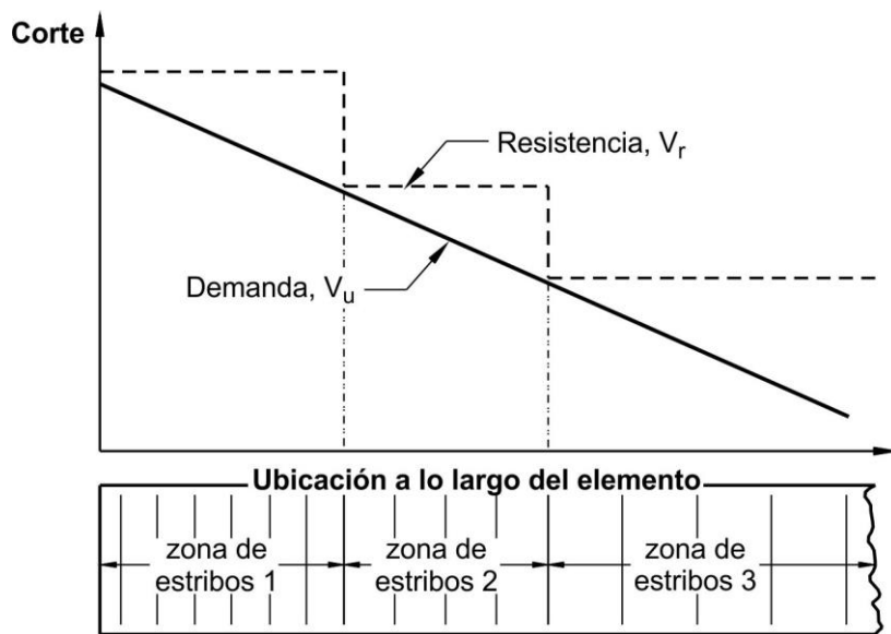
Figura C 5.8.3.2-1. Diseño al corte tradicional
