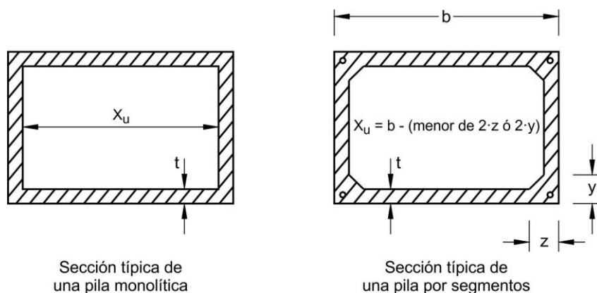
Figura C 5.7.4.7.1-1. Definición de X_u
