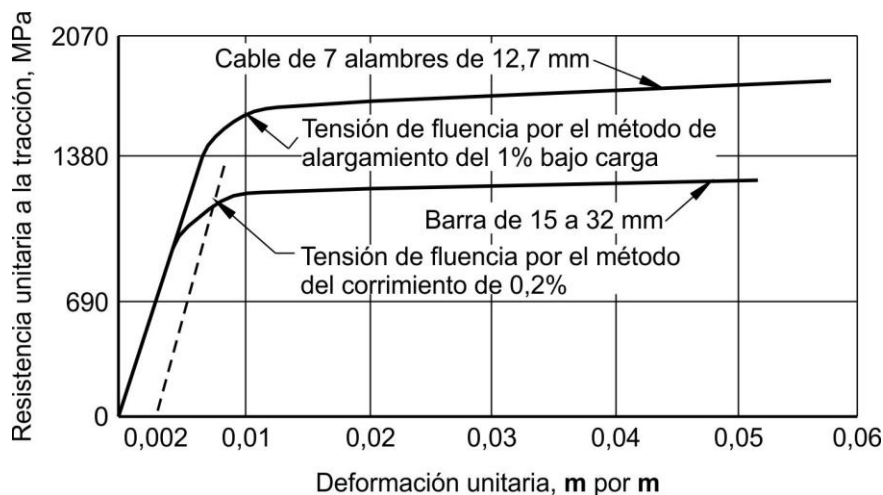
Figura C 5.4.4.2-1. Típica curva tensión-deformación para los aceros de pretensado
