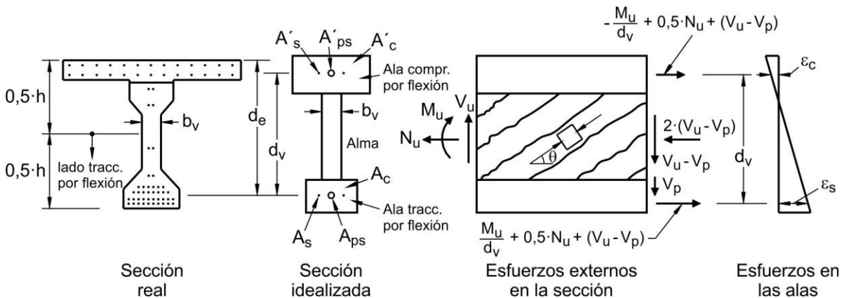
Figura C 5.8.3.4.2-3. Procedimiento de cálculo más preciso para determinar \varepsilon_s
