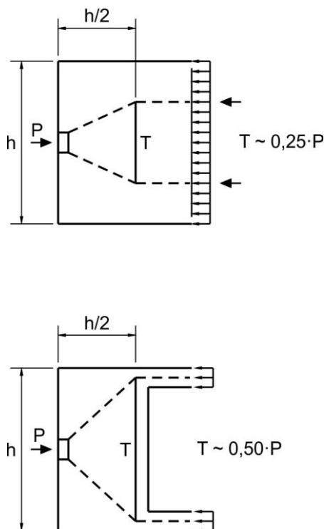
Figura C 5.10.9.6.1-1. Efecto de las discontinuidades en la zona de anclaje
