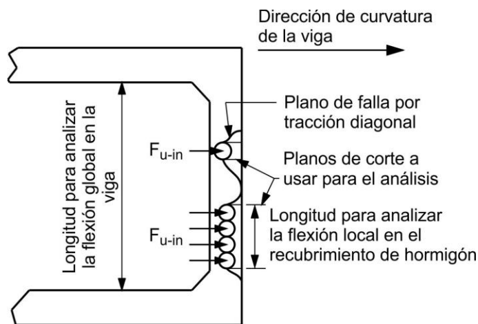
Figura C 5.10.4.3.1a-2. Solicitaciones en el plano en vigas curvas provocadas por cables curvos en el plano horizontal
