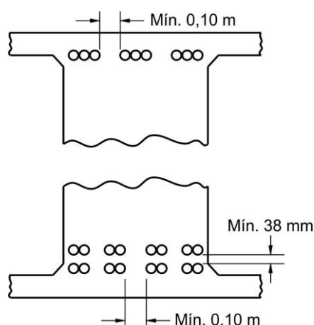
Figura C 5.10.3.3.2-1. Ejemplos de disposiciones aceptables para vainas rectas (no curvas) en el plano horizontal
