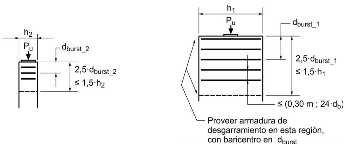
Figura C 5.10.9.3.2-1. Disposición de la armadura de desgarramiento
