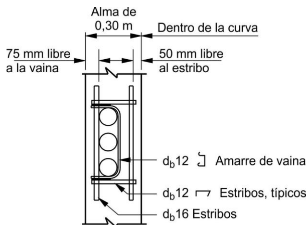
Figura C 5.10.4.3.1b-1. Detalle de estribo abierto típico y amarre de vainas
