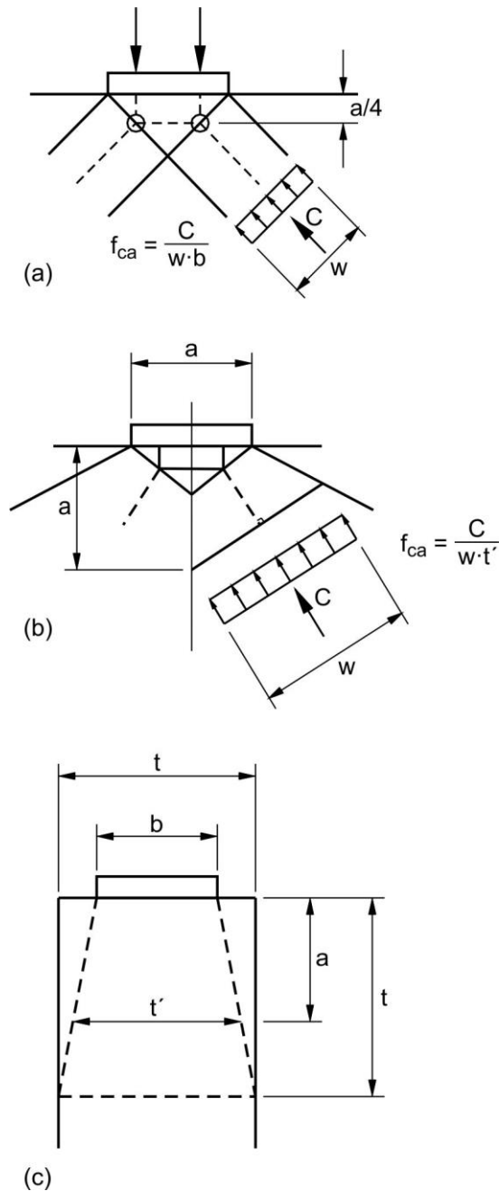
Figura C 5.10.9.4.2-1. Secciones críticas para nodos y bielas comprimidas
