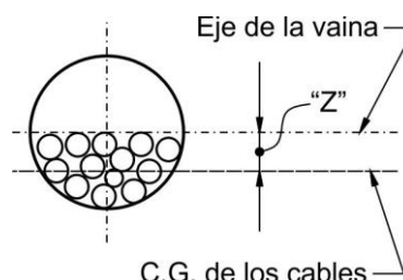
Figura C 5.9.1.6-1. Posición del cable dentro de la vaina
