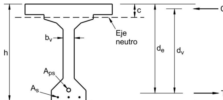
Figura C 5.8.2.9-1. Ilustración de los términos b_v y d_v
