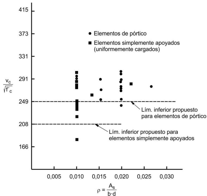
Figura C 5.14.5.3-1. Resultados de ensayos de alcantarillas
