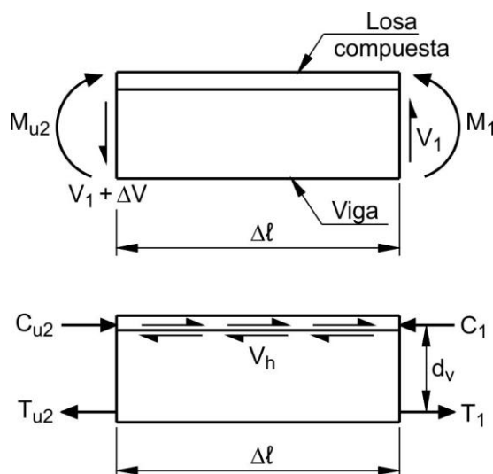
Figura C 5.8.4.2-1. Diagramas de cuerpo libre
