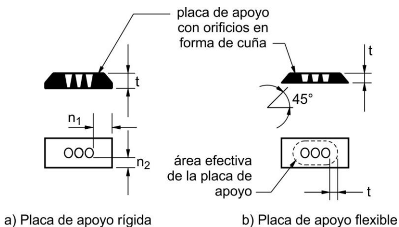
Figura C 5.10.9.7.2-3. Área efectiva de la placa de apoyo para dispositivos de anclaje sin placa de acuñaamiento separada
