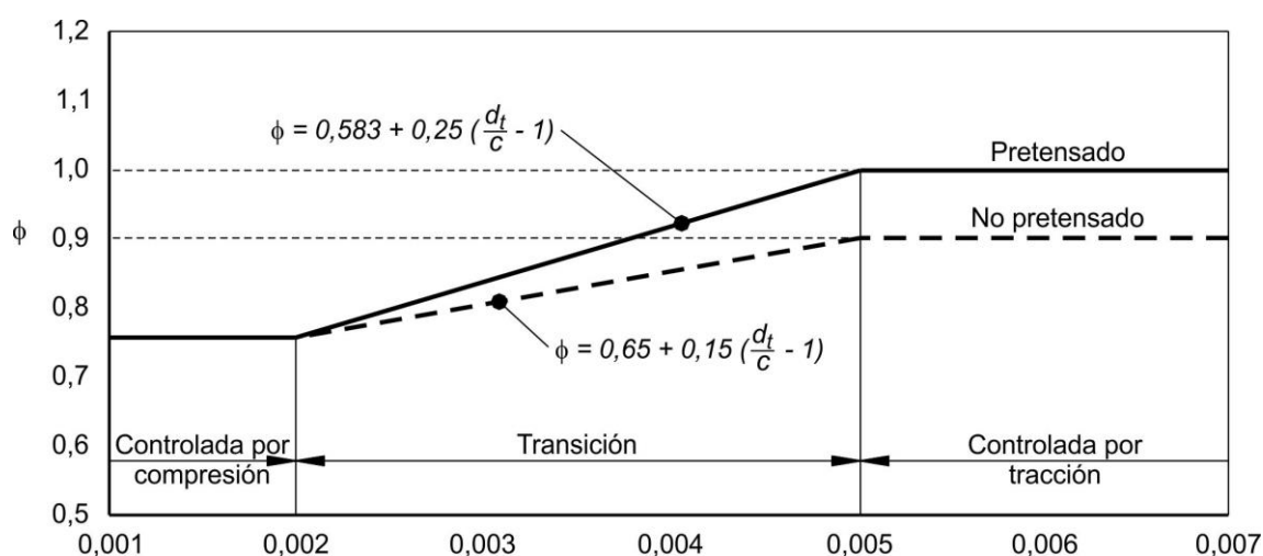
Figura C 5.5.4.2.2-1. Variación de \phi en función de la deformación unitaria neta por tracción \varepsilon_t y d_t/c para armadura f_y = 420 MPa y para acero de pretensado
