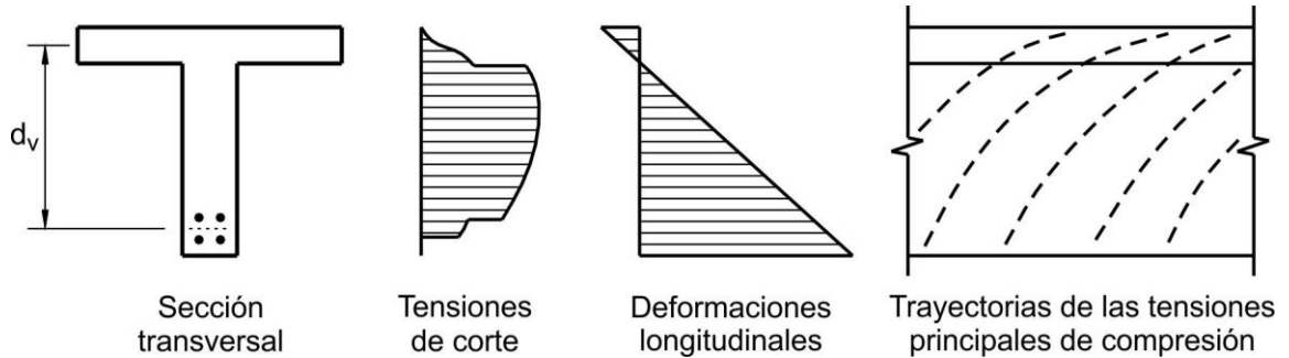
Figura C 5.8.3.4.2-1. Análisis seccional detallado para determinar la resistencia al corte de acuerdo con el artículo 5.8.3.1.
