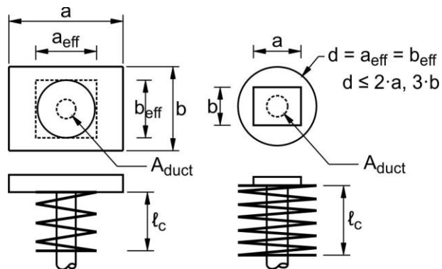
Figura C 5.10.9.6.2-3. Área de apoyo efectiva
