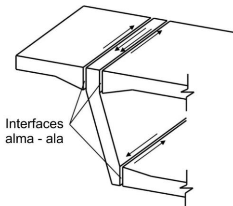
Figura C 5.8.4.1-1. Transferencia de corte longitudinal entre las alas y las almas de los puentes viga tipo cajón
