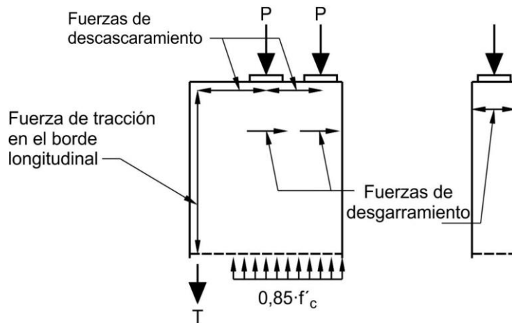
Figura C 5.10.9.3.2-3. Fuerzas de tracción en los bordes
