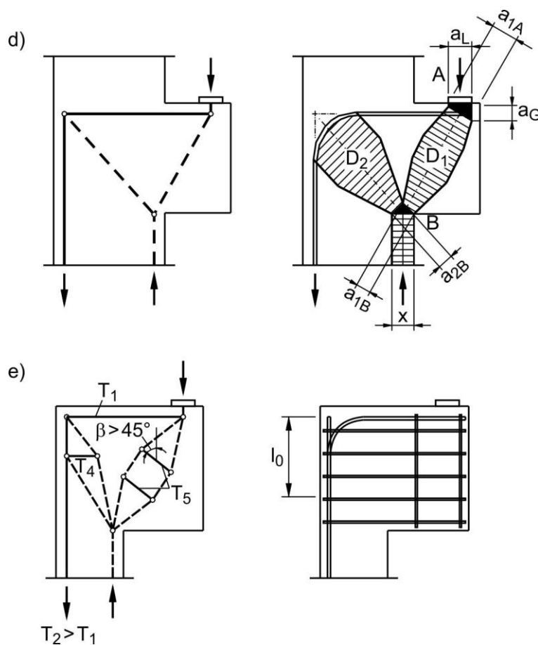
Figura C 5.13.2.4.1-1 (Cont.). Diferentes condiciones de apoyo que conducen a diferentes modelos de bielas y tirantes y diferentes disposiciones de armadura en ménsulas cortas y vigas con resaltos horizontales (Schlaich et al., 1987)
