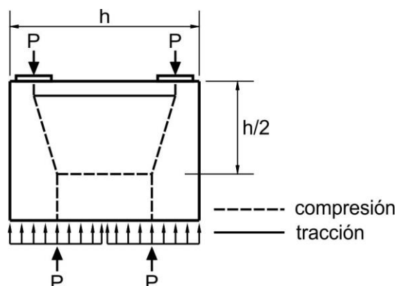
Figura C 5.10.9.3.2-2. Recorrido de las fuerzas para el caso de múltiples anclajes
