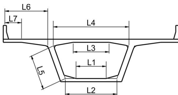
Figura C 5.9.4.2.1-1. Longitudes sugeridas a considerar
