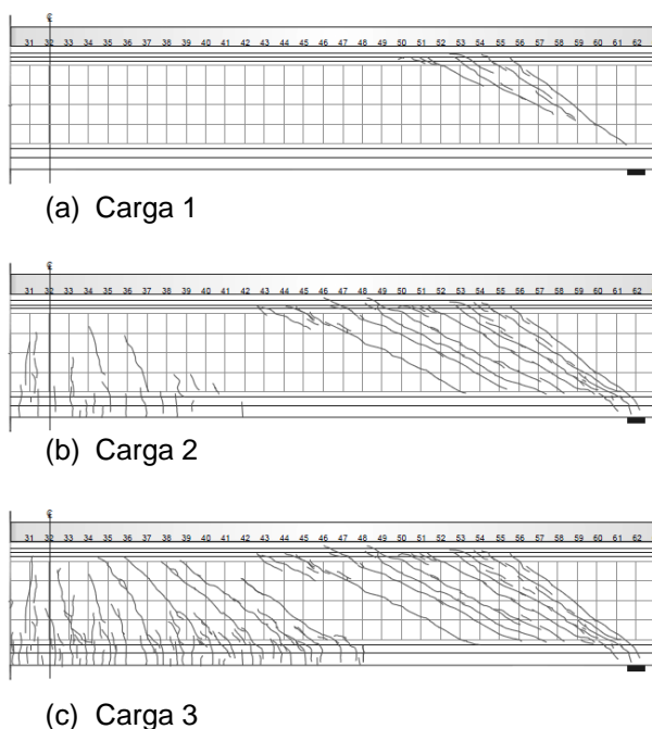
Figura C 5.8.3.4.3-1. Desarrollo de fisuración por corte en una viga en I uniformemente cargada con cargas crecientes; Carga 1 < Carga 2 < Carga 3
